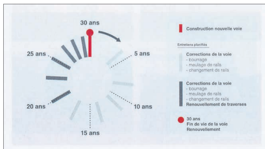
Le cycle de vie d'une voie ferrée
