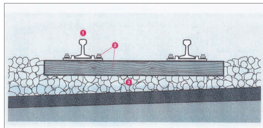
1. Le rail 2. Les attaches et les traverses 3. Le ballast
